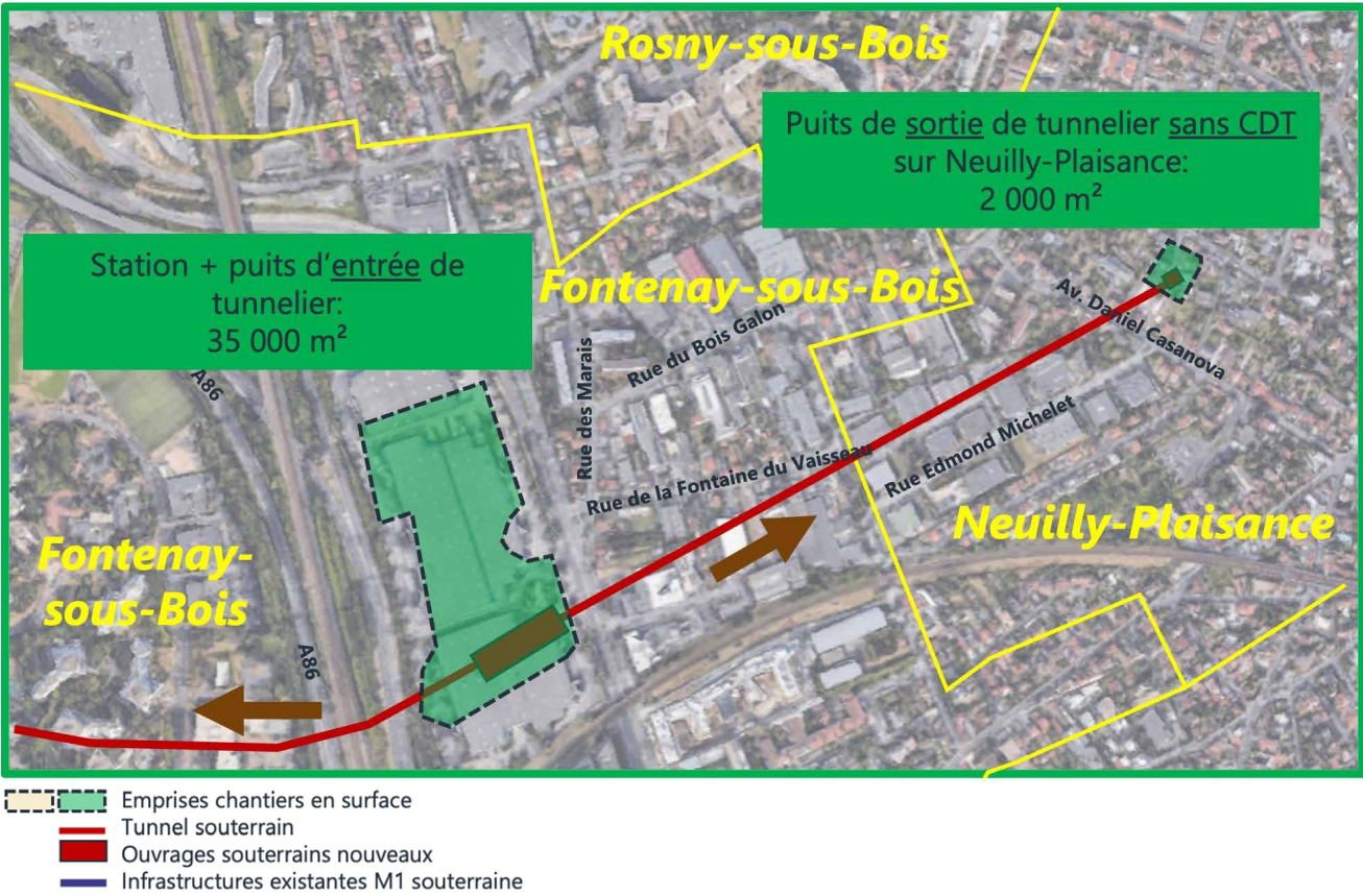
↓ Val de Fontenay, variante C – Emprises chantiers
