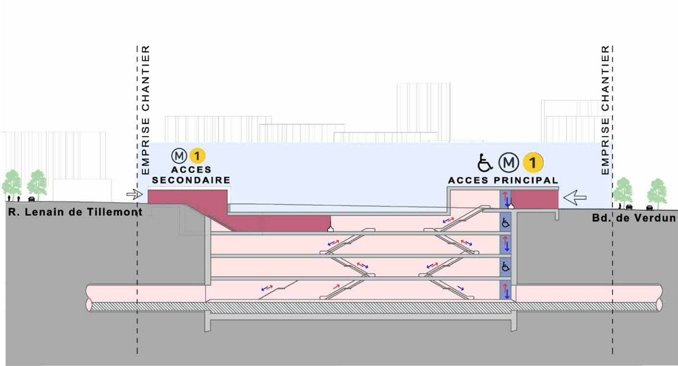
↓ Coupe de principe – Station Grands Pêchers, nouveau principe d'insertion des accès : intégration à un projet urbain
