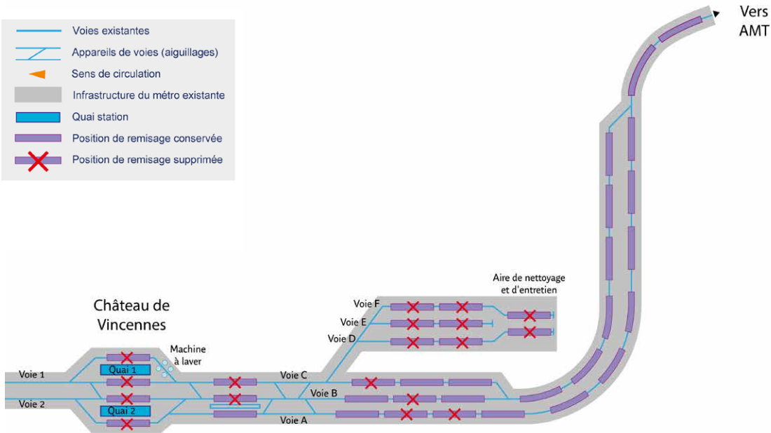
Schéma représentant la configuration de l'arrière-gare existante de Château de Vincennes, les places de garage des rames qui seraient conservées et supprimées avec le projet
