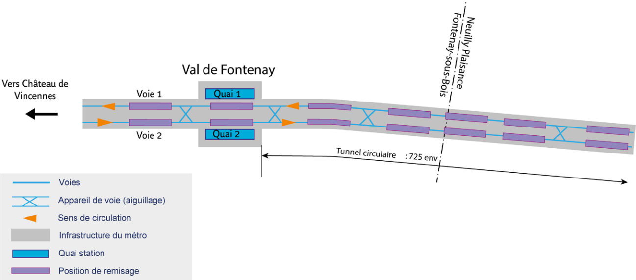
↓ Synoptique du remisage dans la nouvelle arrière-gare de Val de Fontenay – Variante C
