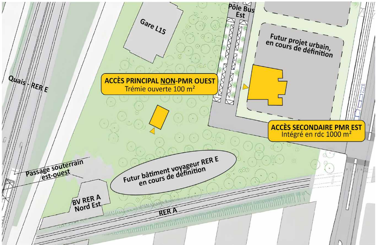
↓ Principe d'insertion alternatif : scénario n°2
