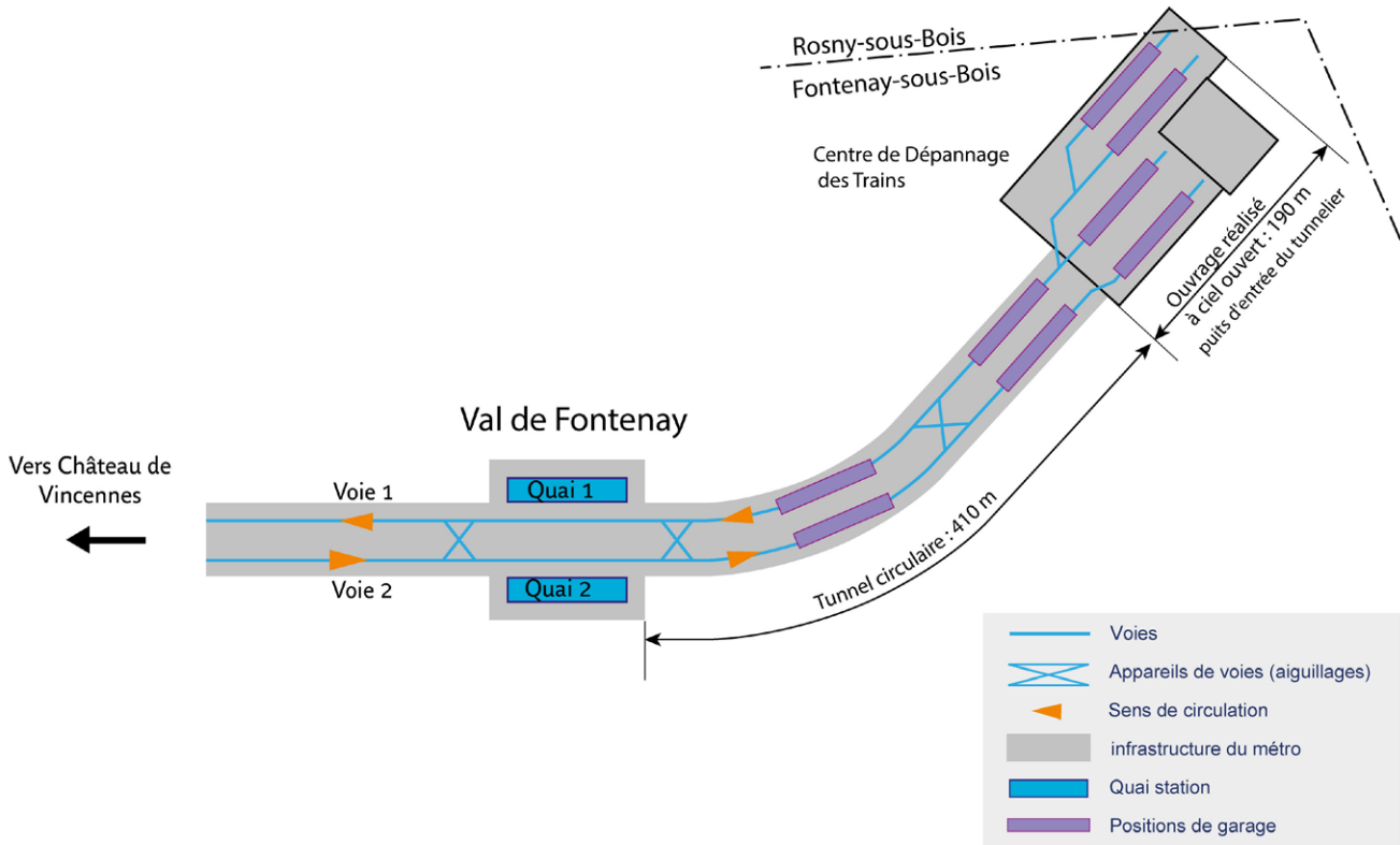
↓ Synoptique du remisage dans la nouvelle arrière-gare de Val de Fontenay – Variante A
