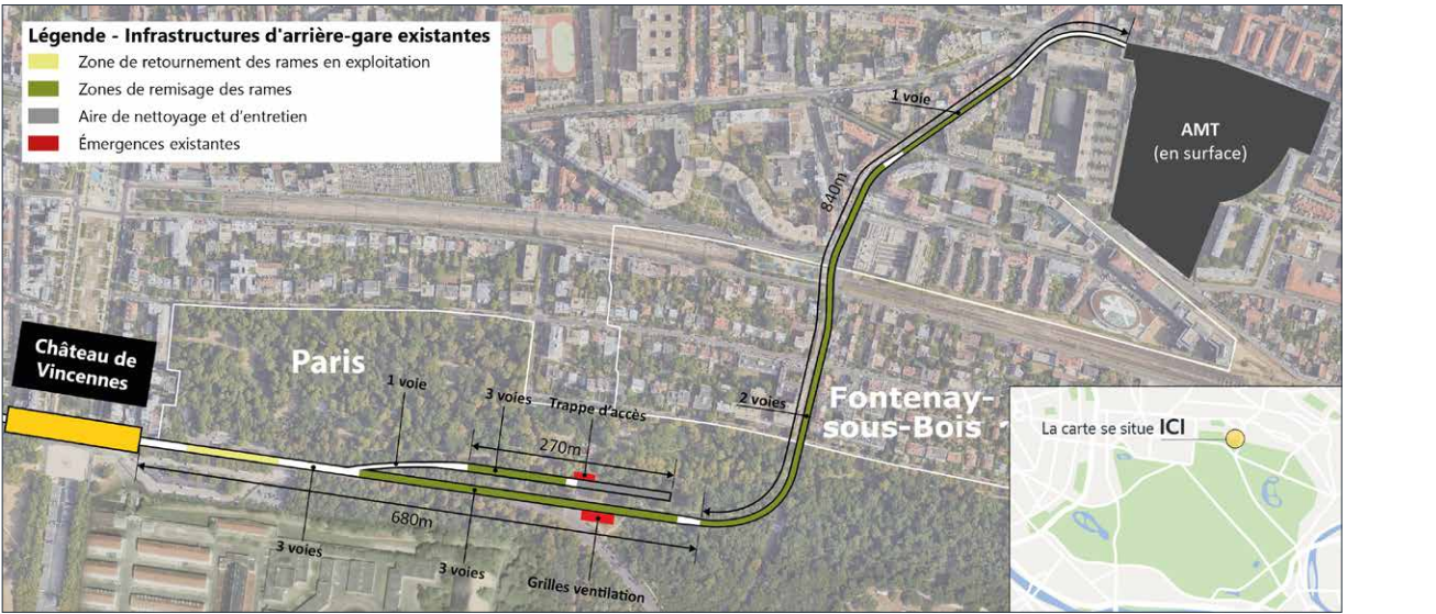
↓ Disposition de l'arrière-gare actuelle de Château de Vincennes et liaison vers les ateliers de Fontenay-sous-Bois
