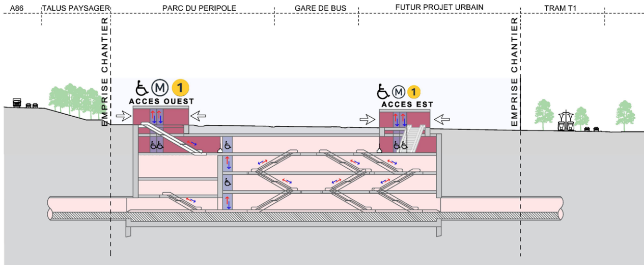
Principe d'insertion alternatif de la station Val de Fontenay : scénario n°1
