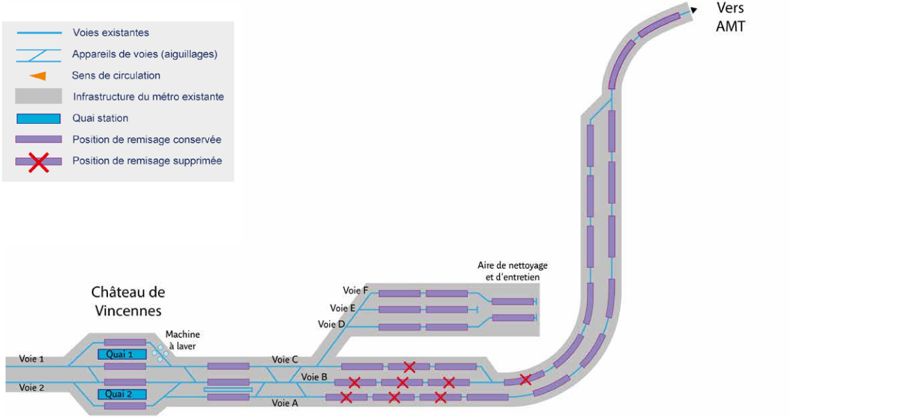
Schéma représentant la configuration de l'arrière-gare existante de Château de Vincennes, les places de garage des rames qui seraient conservées et supprimées avec le projet
