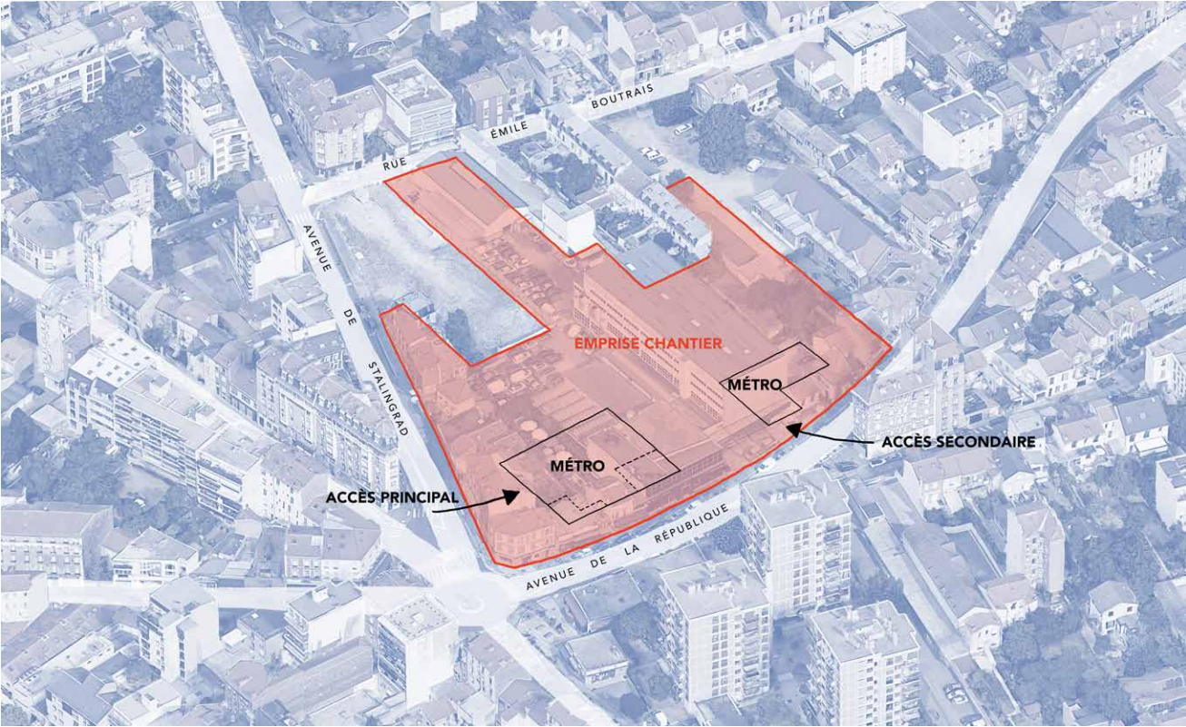
↓ Vue en plan de l'emprise chantier pour la station Les Rigolots
