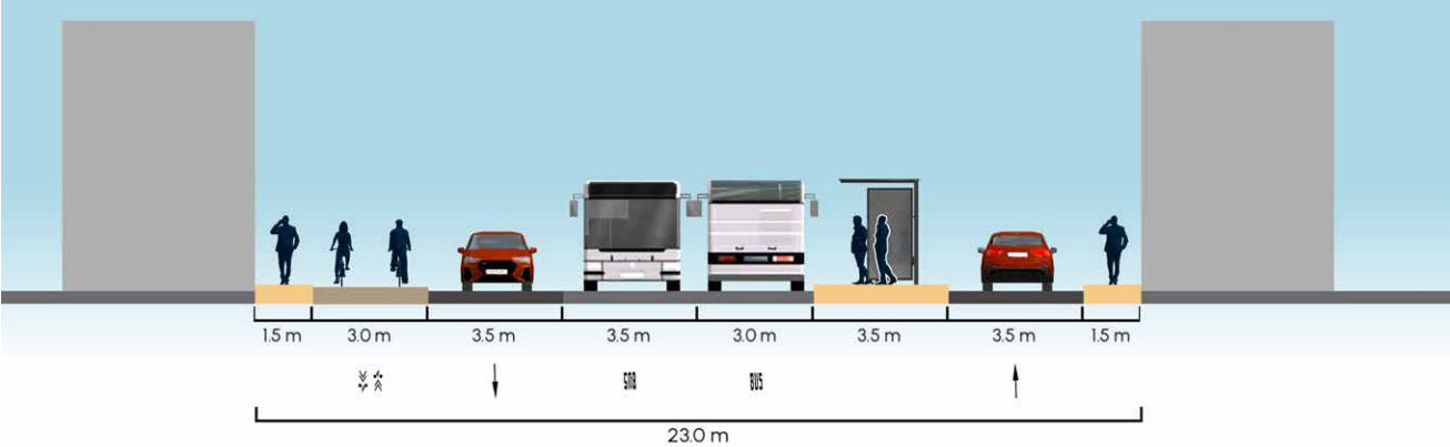
↓ Largeur minimale pour le cas n°2-A en station
