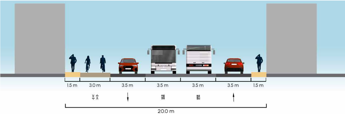
↓ Largeur minimale pour le cas n°2-A en section courante
