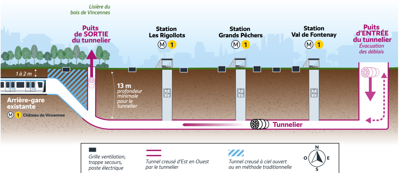
↓ Schéma de creusement du tunnel (non à l'échelle)
