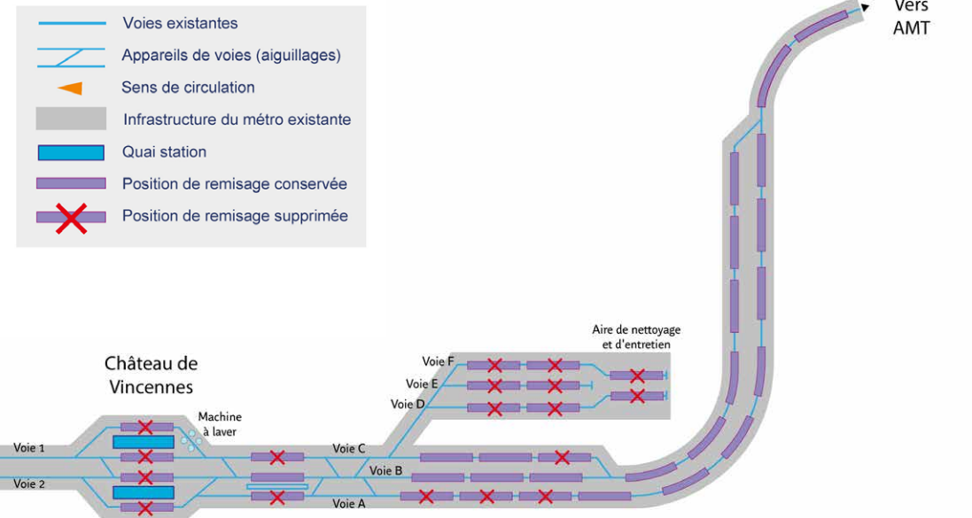
Schéma représentant la configuration de l'arrière-gare existante de Château de Vincennes, les places de garage des rames qui seraient conservées et supprimées avec le projet
