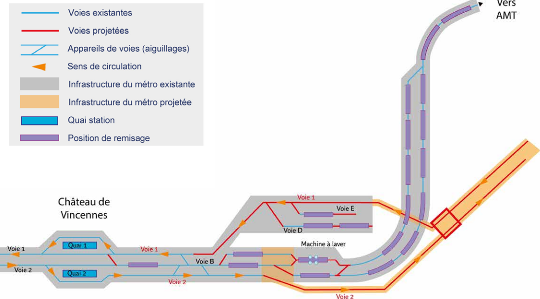
Schéma représentant la configuration de l'arrière-gare de Château de Vincennes et les places de garage des rames - situation avec le projet
