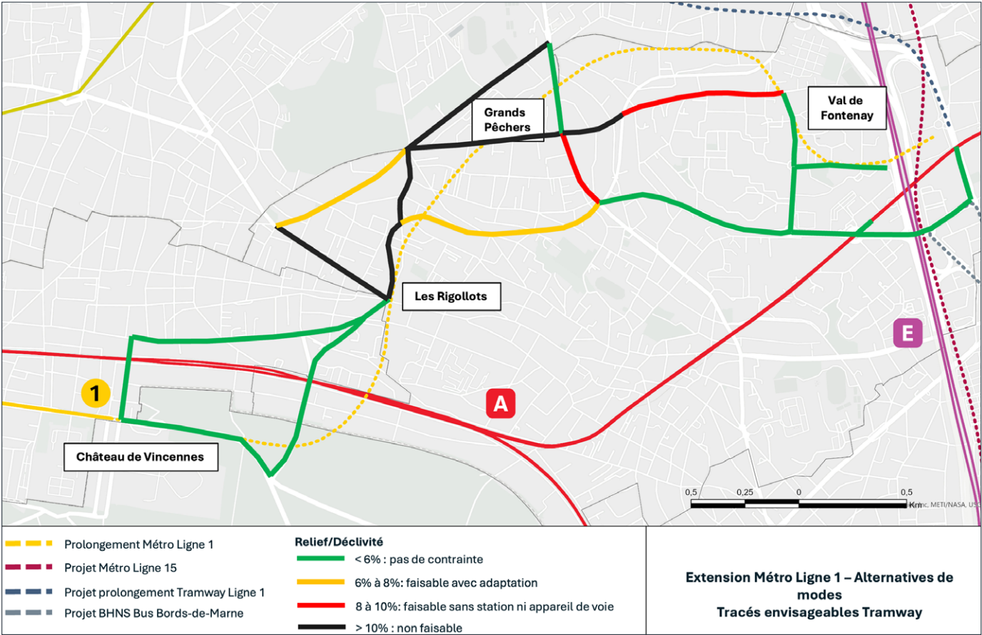
↑ Pentes par tronçon sur les itinéraires pré-identifiés
